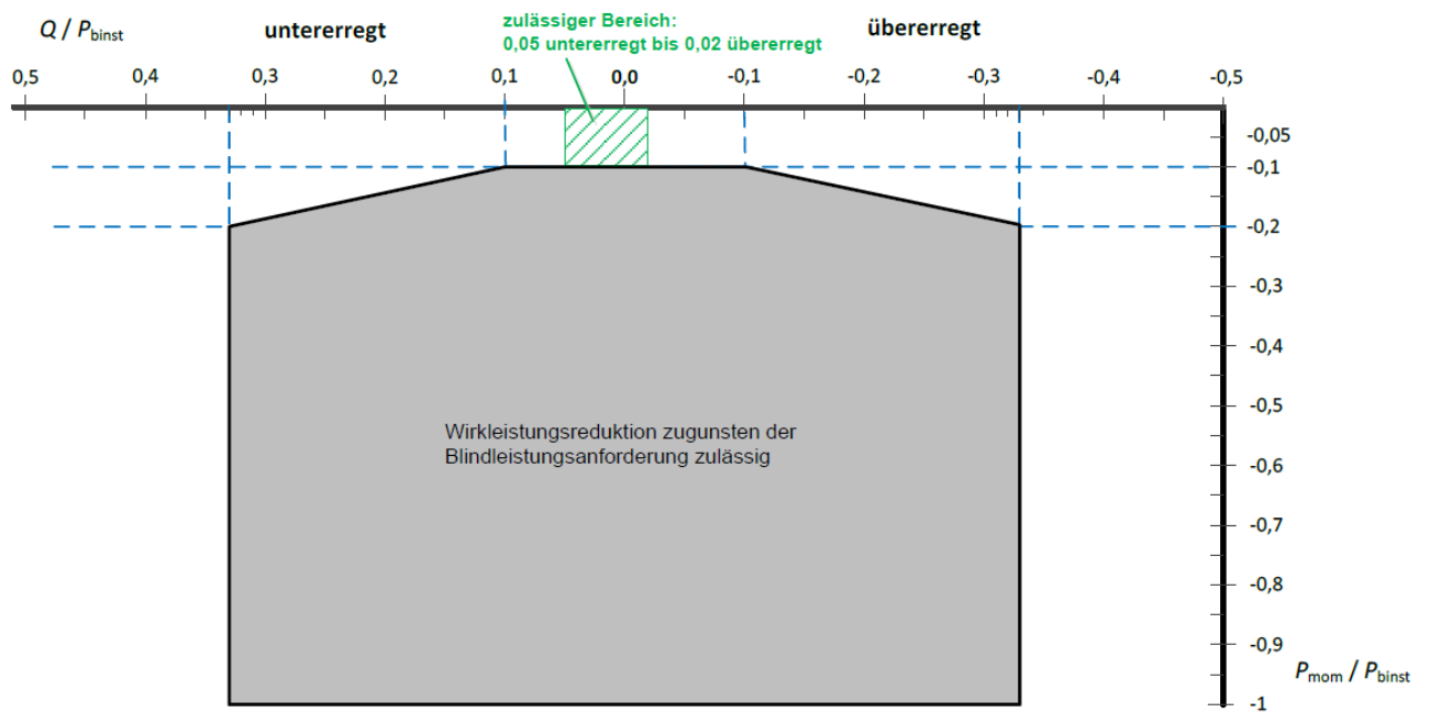
Bild 1 Geforderter Stellbereich der Blindleistung für Erzeugungsanlagen mit P_{Amax} \geq 135 kW (VDE-AR-N 4110)
